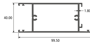
DOOR - BOTTOM SECTION NO. : 812659 Weight / Mtr : 1.298
