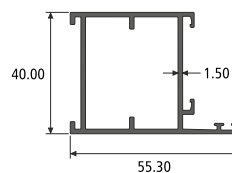
DOOR FRAME SECTION NO. : 819022 Weight / Mtr : 0.783
