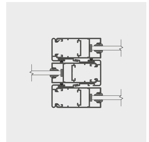
29mm FLYMESH
