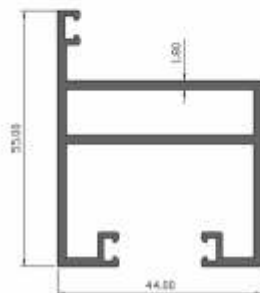
DOOR PROFILE
